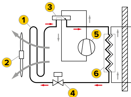
Rys. 2. Tryb grzania w pompie ciepła
