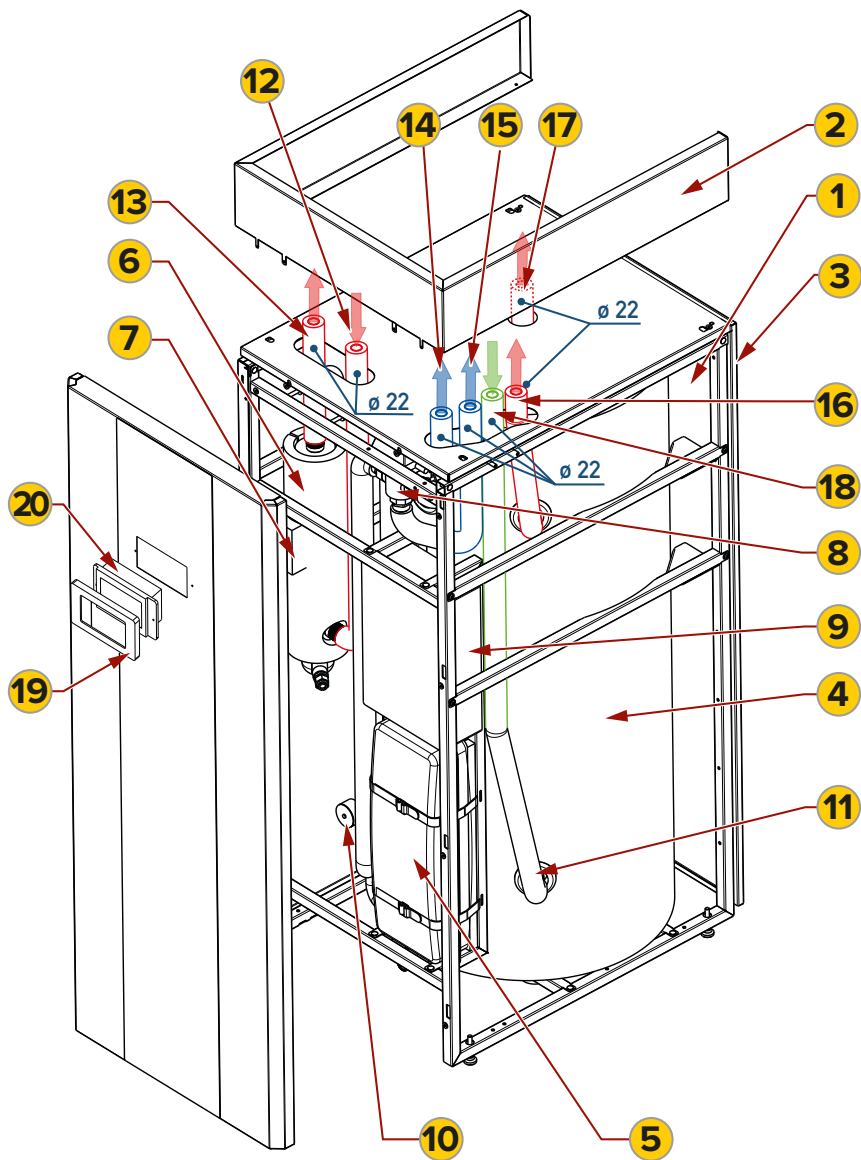
Rys. 18. Schemat wieży hydraulicznej
